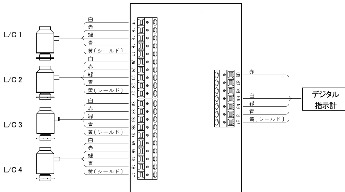
ジャンクションボックス内部端子台 接続図
